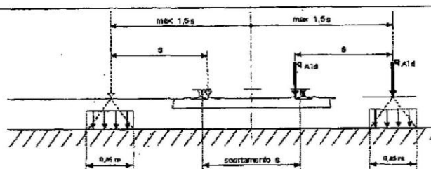
Fig. a - Deragliamento sopra il ponte - caso 1
