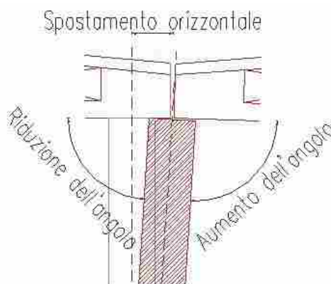
Schematizzazione del comportamento del giunto trave-pilastro
