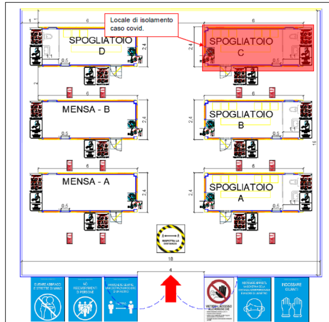
Planimetria del campo base con individualizzazione dello spogliatoio ad uso
